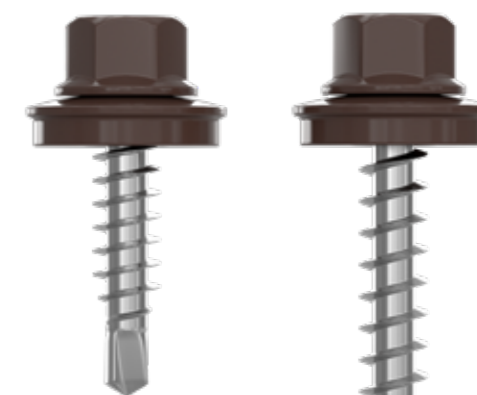
Șurub coasere (metal-metal) 4,8 x 20 mm
